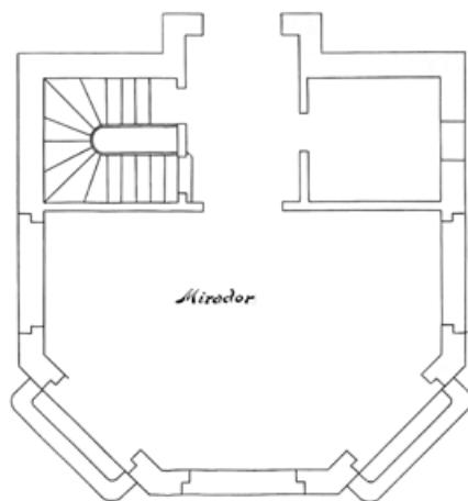
Escala 1:50
